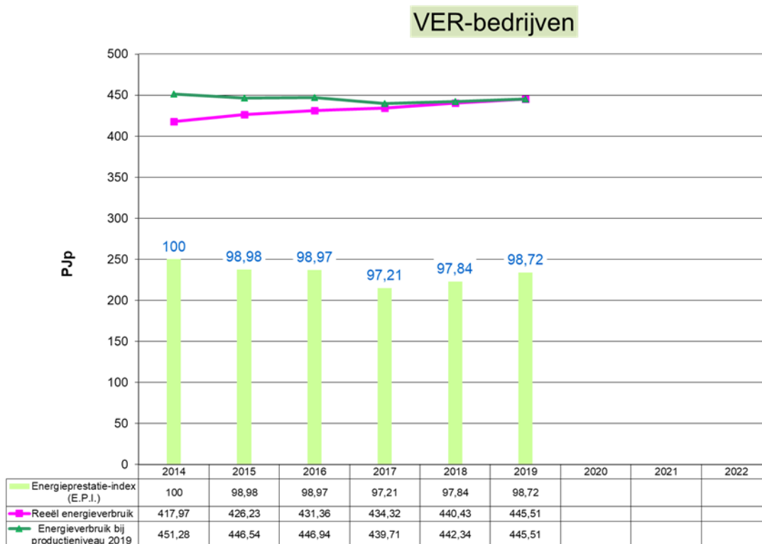
Grafiek 27: Evolutie 2014 – 2019 van het energieverbruik en de E.P.I. voor de VER-bedrijven
