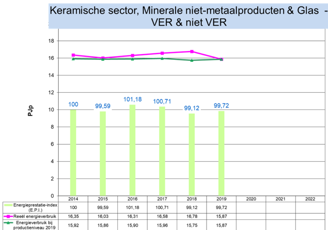
Grafiek 45: Evolutie 2014 – 2019 van het energieverbruik en de E.P.I. voor Keramische sector, Minerale niet-metaalproducten & Glas (VER en niet VER-bedrijven)
