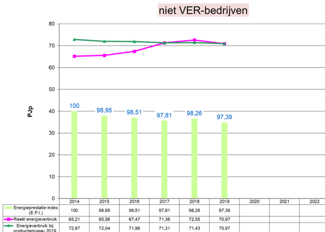
Grafiek 28: Evolutie 2014 – 2019 van het energieverbruik en de E.P.I. voor de niet VER-bedrijven
