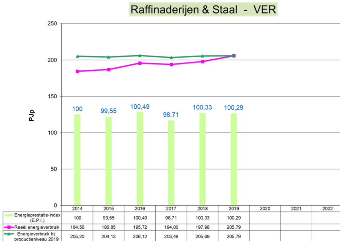
Grafiek 32: Evolutie 2014 – 2019 van het energieverbruik en de E.P.I. voor Raffinaderijen & Staal (VER-bedrijven)
