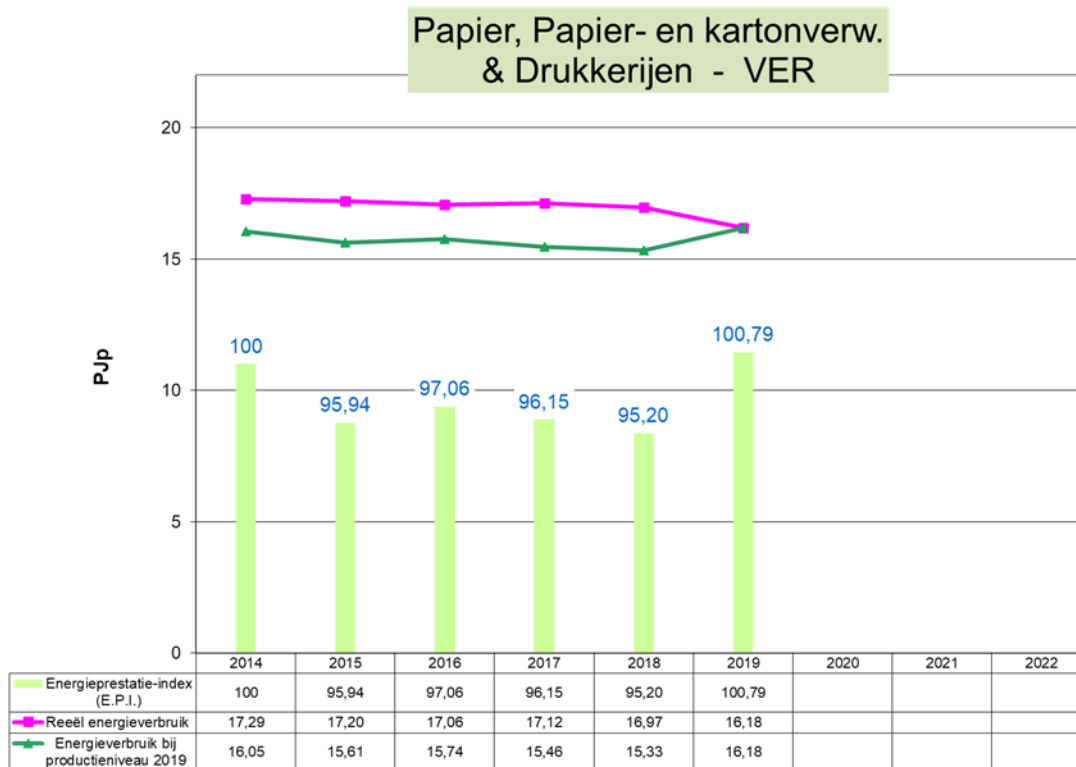
Grafiek 34: Evolutie 2014 – 2019 van het energieverbruik en de E.P.I. voor Papier, Papier- en kartonverwerking & Drukkerijen (VER-bedrijven)
