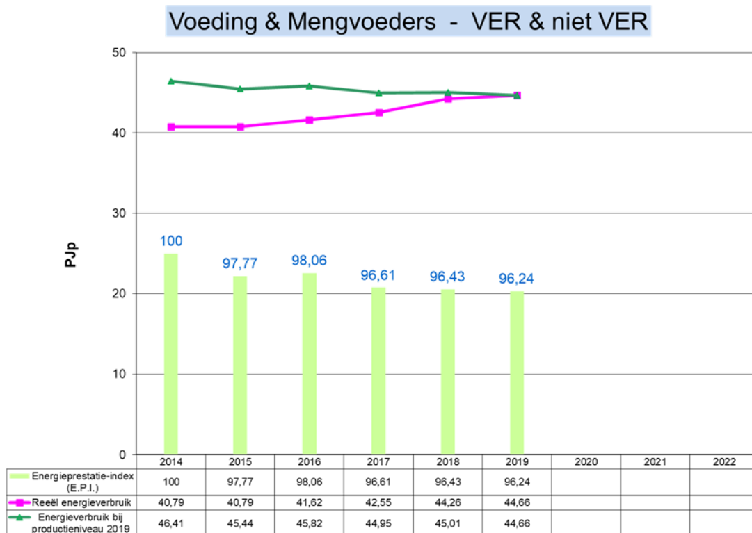
Grafiek 36: Evolutie 2014 – 2019 van het energieverbruik en de E.P.I. voor Voeding & Mengvoeders (VER en niet VER-bedrijven)
