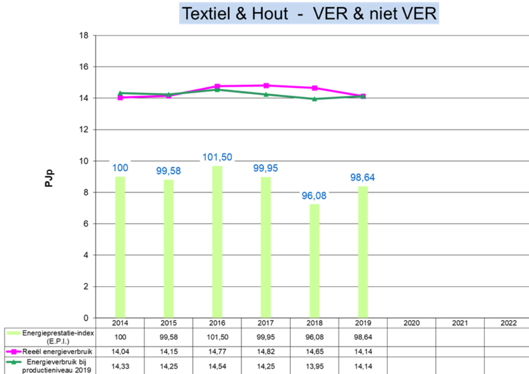
Grafiek 42: Evolutie 2014 – 2019 van het energieverbruik en de E.P.I. voor Textiel & Hout (VER en niet VER-bedrijven)
