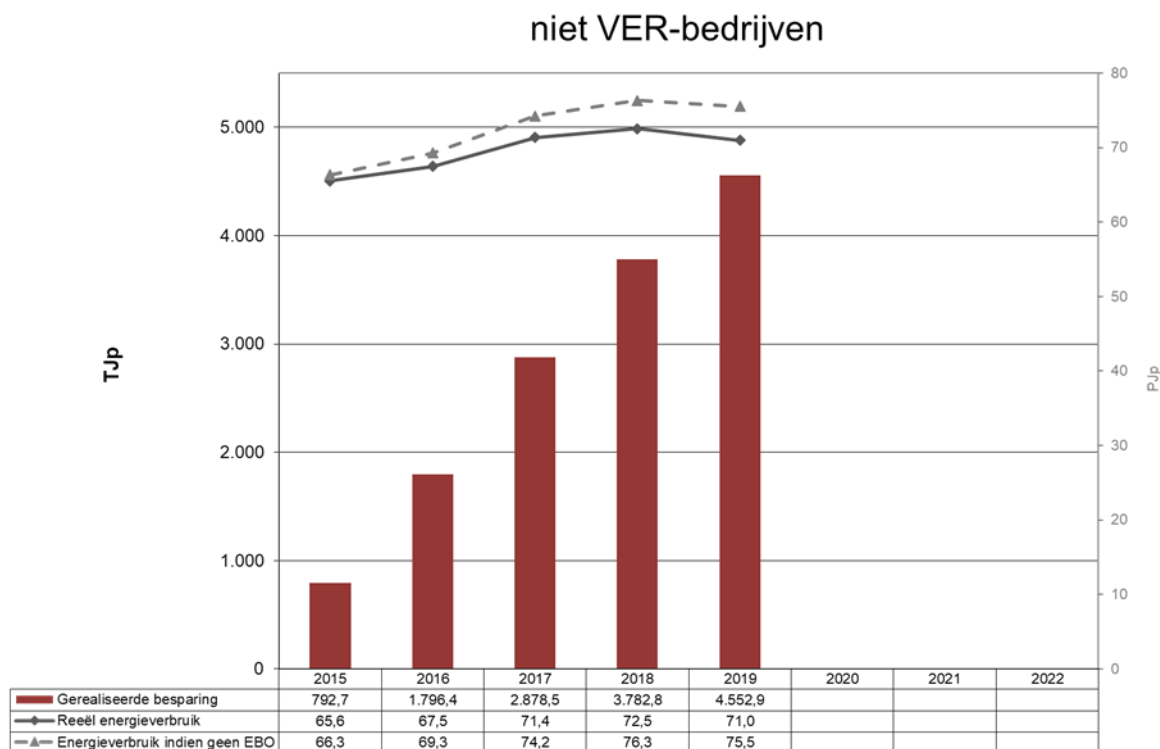
Grafiek 3: Gerealiseerde besparingen (niet VER-bedrijven)
