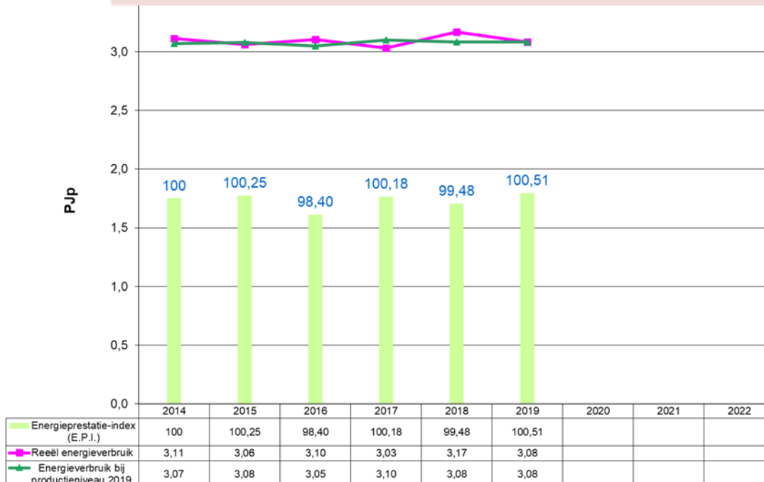
Grafiek 47: Evolutie 2014 – 2019 van het energieverbruik en de E.P.I. voor Keramische sector, Minerale niet-metaalproducten & Glas (niet VER-bedrijven)
