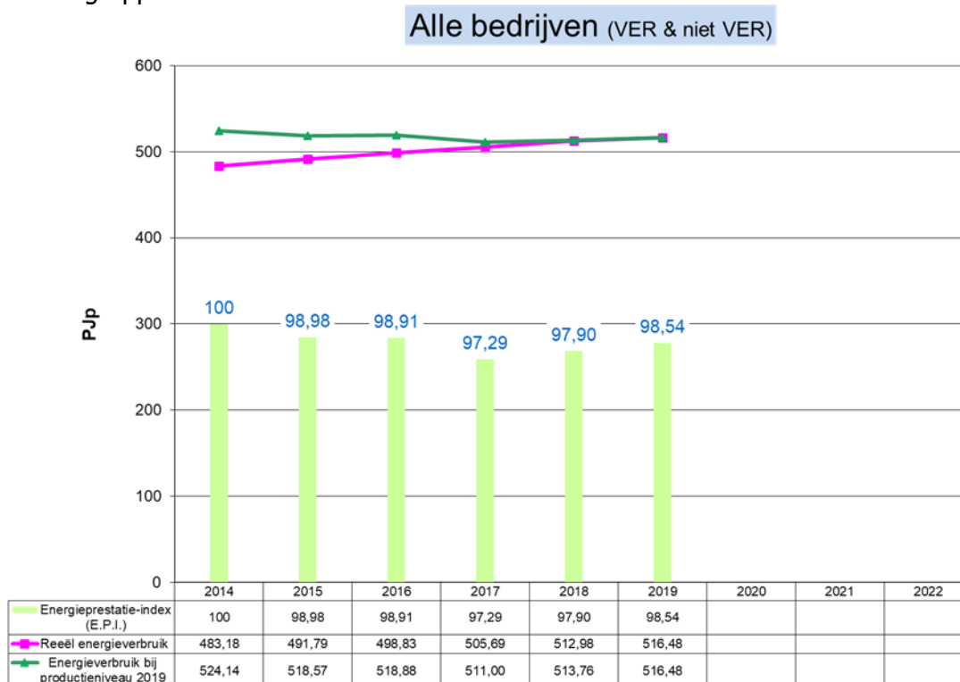
Grafiek 26: Evolutie 2014 – 2019 van het energieverbruik en de E.P.I. voor alle bedrijven
