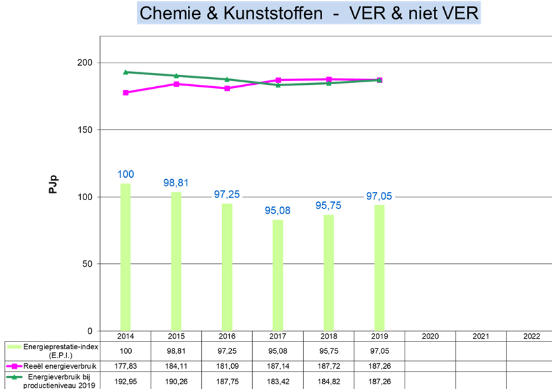
Grafiek 29: Evolutie 2014 – 2019 van het energieverbruik en de E.P.I. voor Chemie & Kunststoffen (VER en niet VER-bedrijven)
