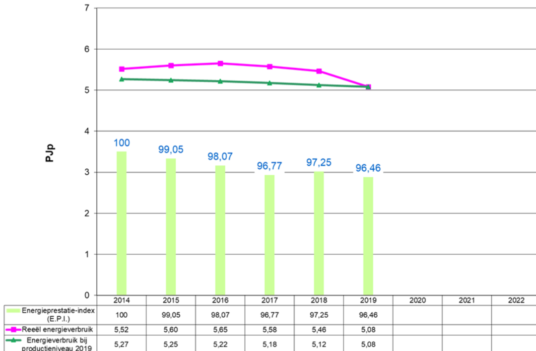
Grafiek 44: Evolutie 2014 – 2019 van het energieverbruik en de E.P.I. voor Textiel & Hout (niet VER-bedrijven)
