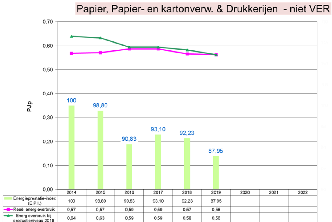
Grafiek 35: Evolutie 2014 – 2019 van het energieverbruik en de E.P.I. voor Papier, Papier- en kartonverwerking & Drukkerijen (niet VER-bedrijven)
