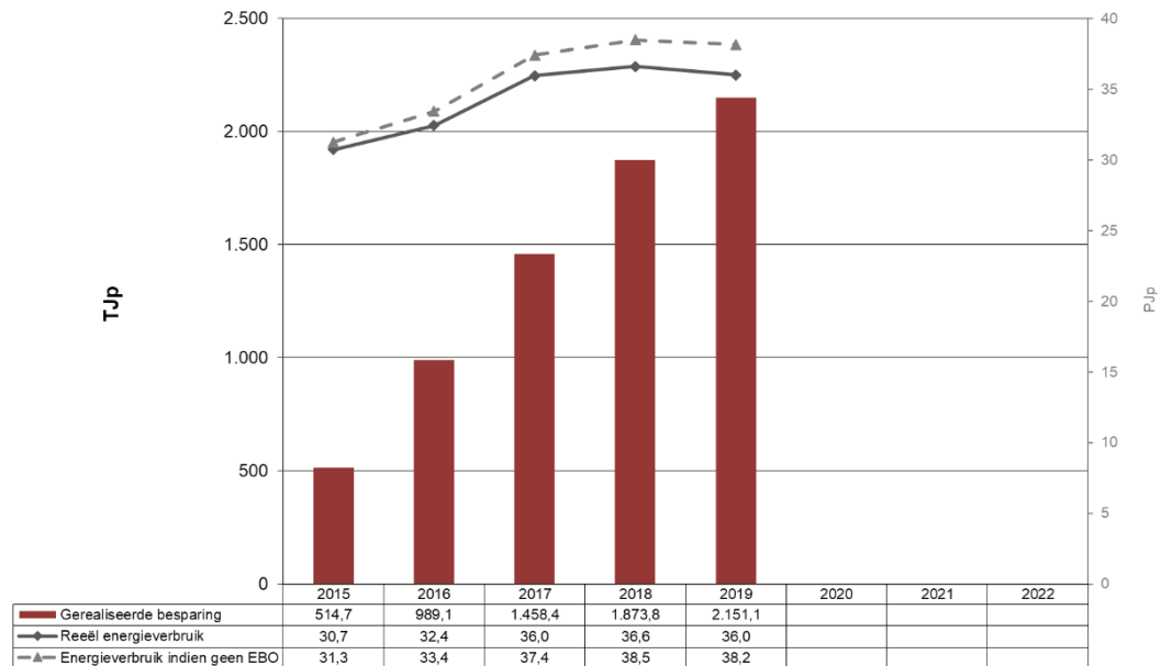
Grafiek 6: Gerealiseerde besparingen Chemie & Kunststoffen (niet VER-bedrijven)
