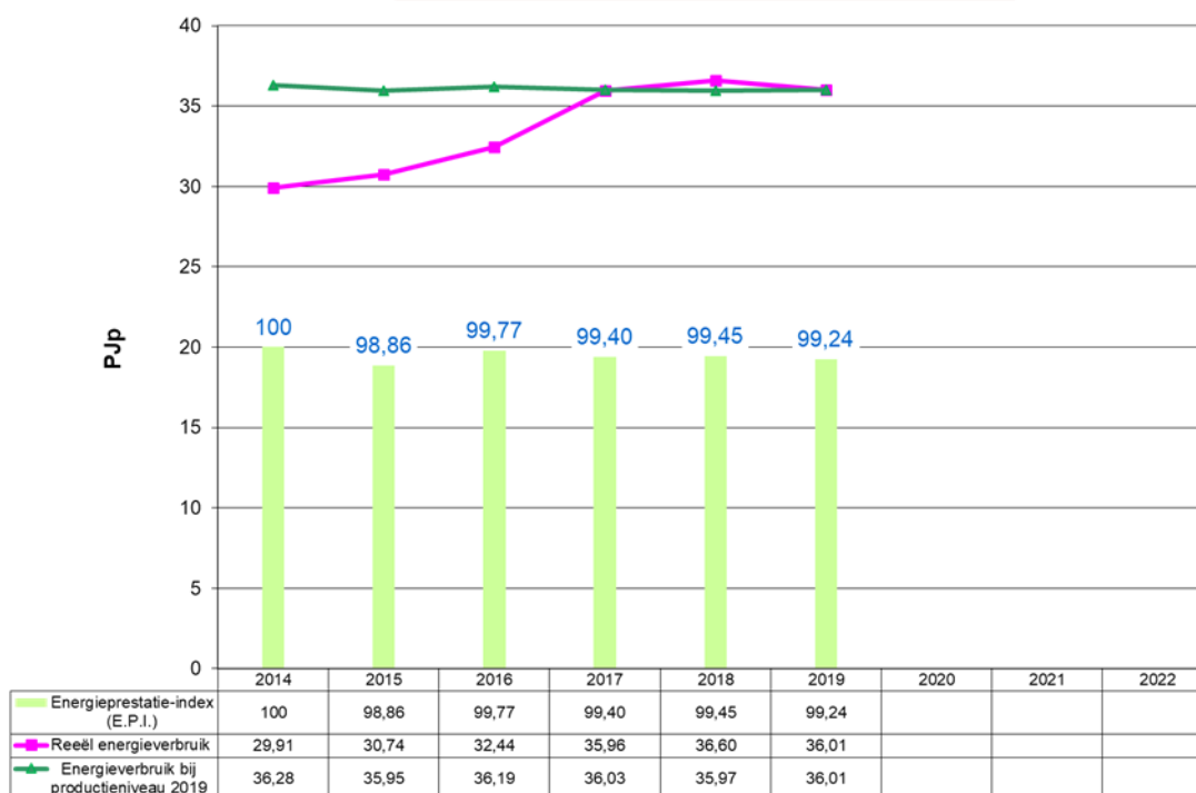
Grafiek 31: Evolutie 2014 – 2019 van het energieverbruik en de E.P.I. voor Chemie & Kunststoffen (niet VER-bedrijven)
