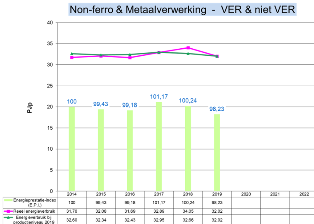
Grafiek 39: Evolutie 2014 – 2019 van het energieverbruik en de E.P.I. voor Non-ferro & Metaalverwerking (VER en niet VER-bedrijven)
