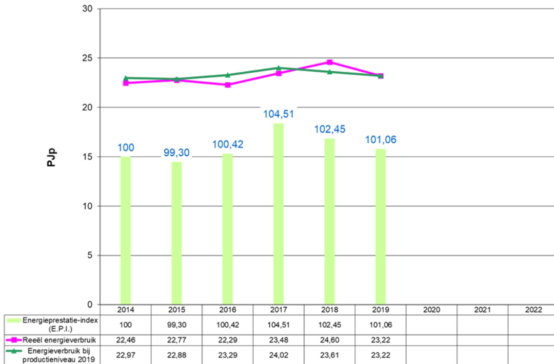
Grafiek 40: Evolutie 2014 – 2019 van het energieverbruik en de E.P.I. voor Non-ferro & Metaalverwerking (VER-bedrijven)
