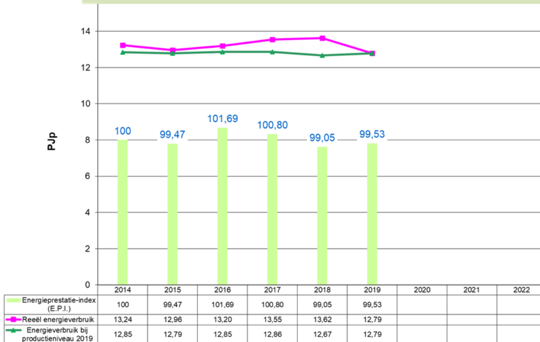
Grafiek 46: Evolutie 2014 – 2019 van het energieverbruik en de E.P.I. voor Keramische sector, Minerale niet-metaalproducten & Glas (VER-bedrijven)
